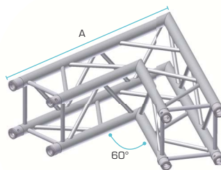
2 WAY CORNER 60°
