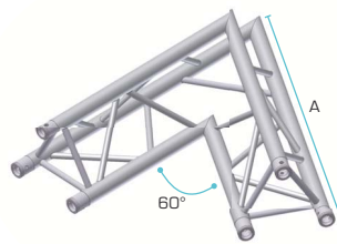
2 WAY CORNER 60°
